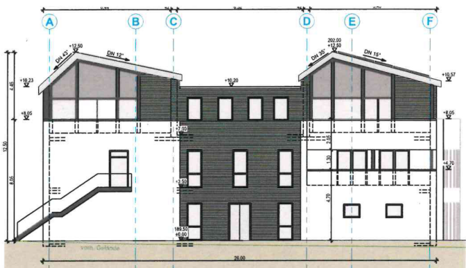
ANSICHT SÜD-WEST
