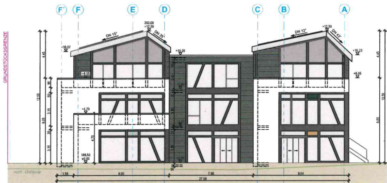
ANSICHT NORD-OST
