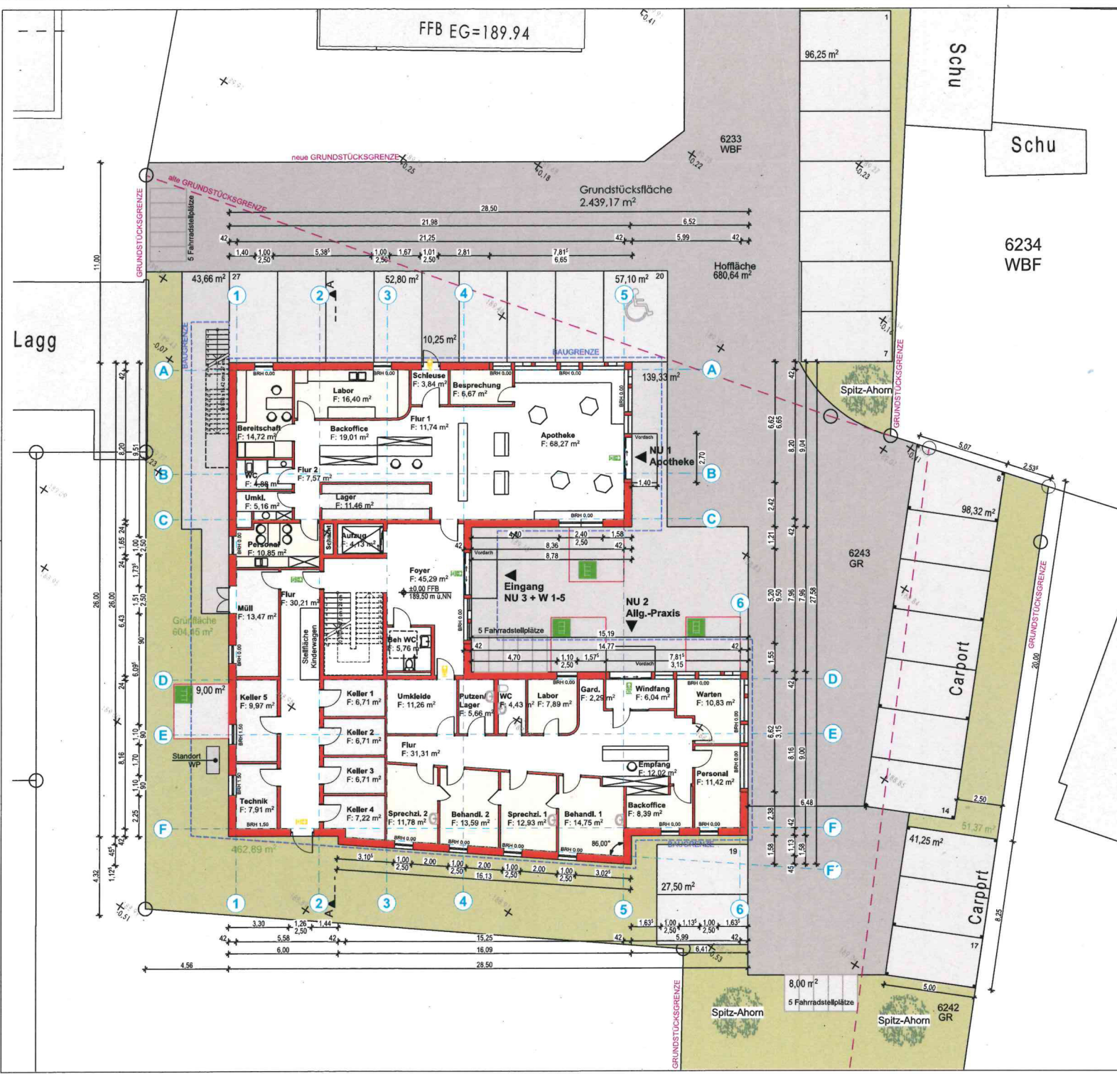
ÜBERSICHT M. 1:500
