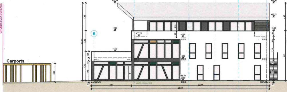
ANSICHT NORD-WEST
