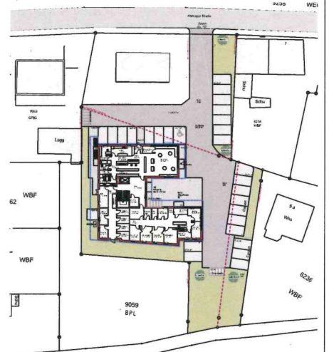
ÜBERSICHT M. 1:500
