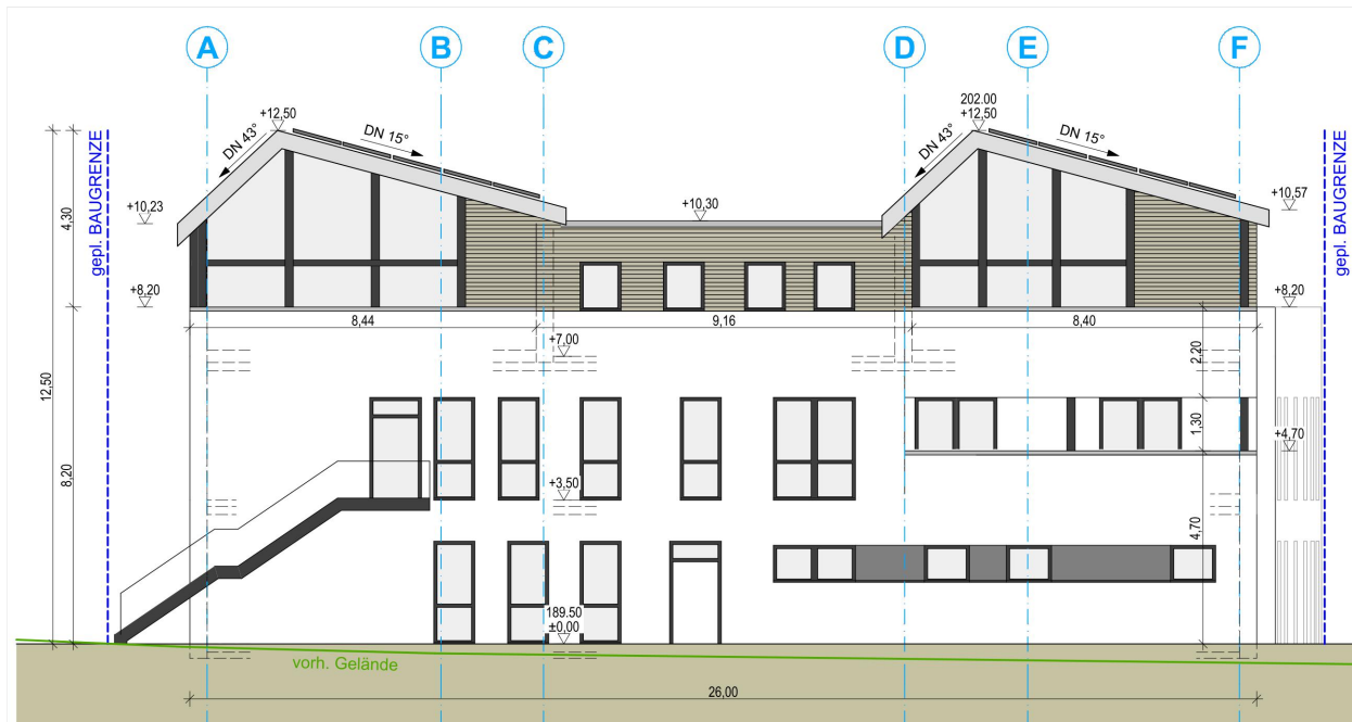
ANSICHT SÜD-WEST
