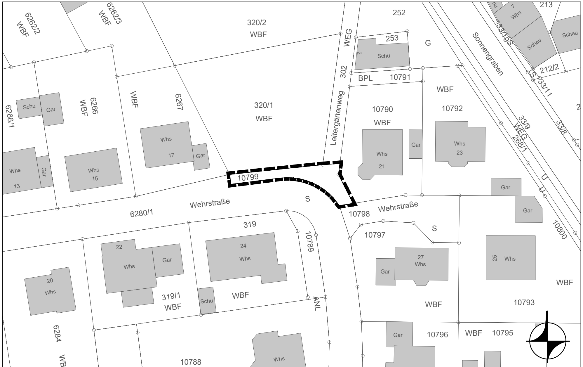
Kürnbach - Bebauungsplan "Beim Friedhof/Leitergärten" - 1. Änderung - Übersichtsplan Geltungsbereich, M 1:500
